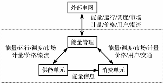
图 1 智能微网信息交互关系 Fig. 1 Information exchange for smart microgrid operation
